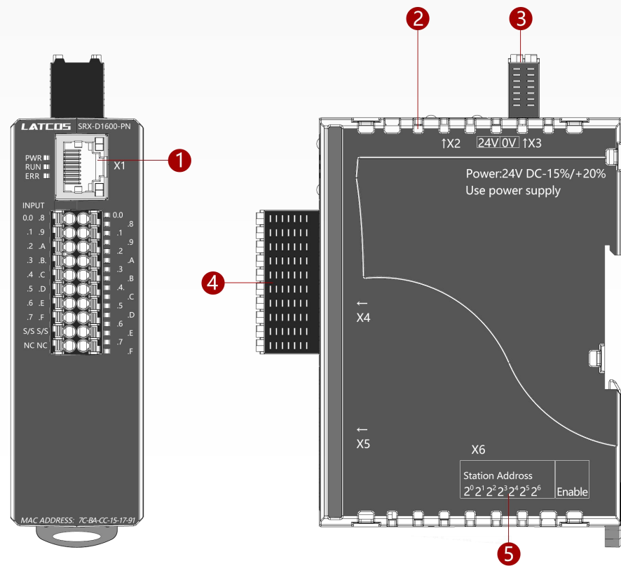
图 3 模块结构图
