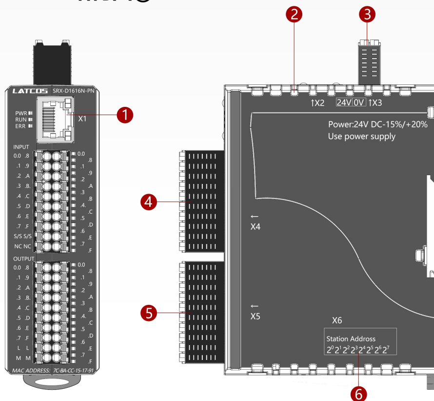
图 4 模块接线图
