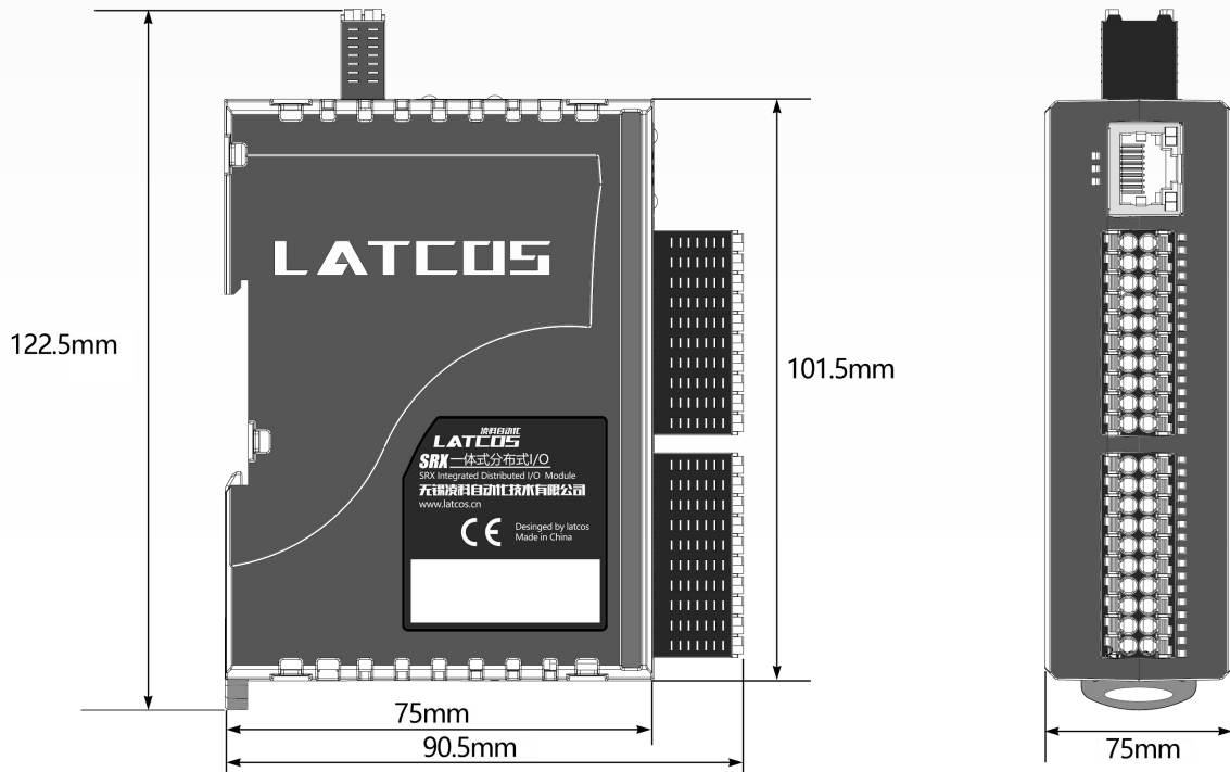
图 1 模块尺寸图
