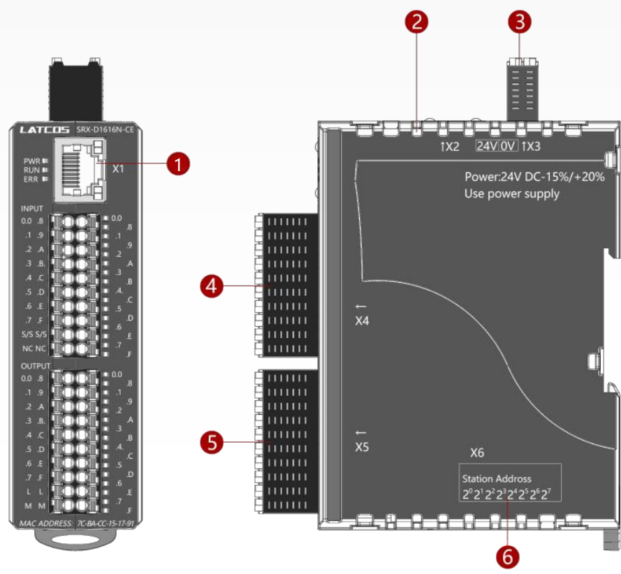
图 4 模块接线图
