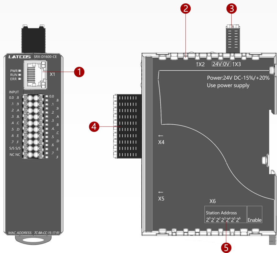
图 3 模块接线图
