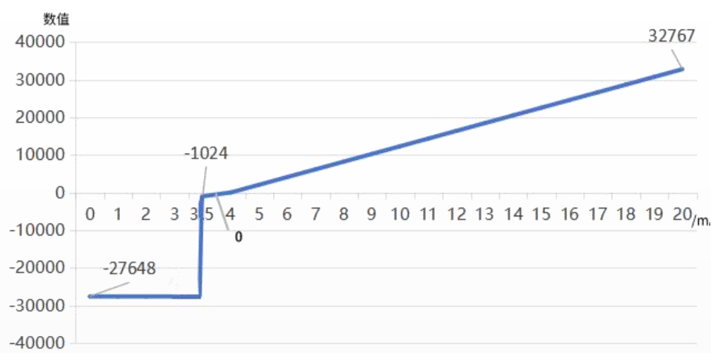
4-20mA电流折线图
