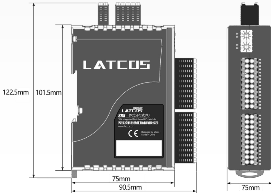
图 1 模块尺寸图
