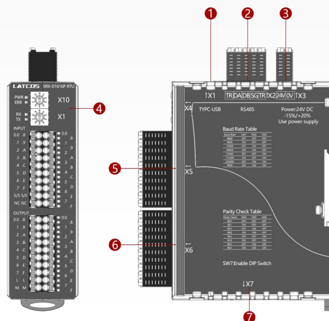
图 4 模块接线图
