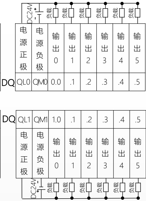
E20C2 数字量 12 点输出模块 NPN 型
