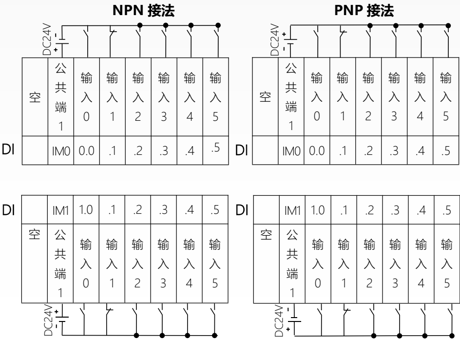
E10C1 数字量 12 点输入模块
