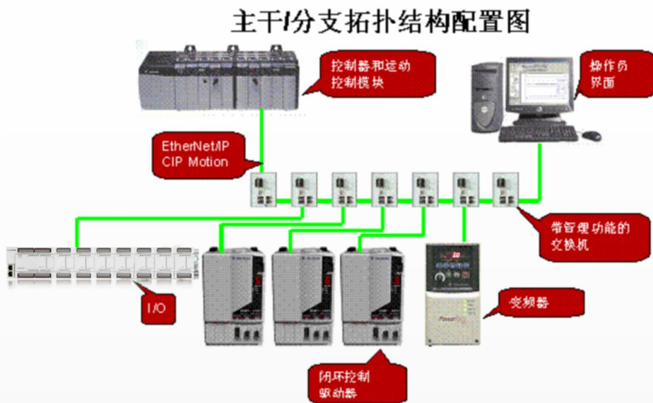
图 3:ETHERNET IP 的网络结构
