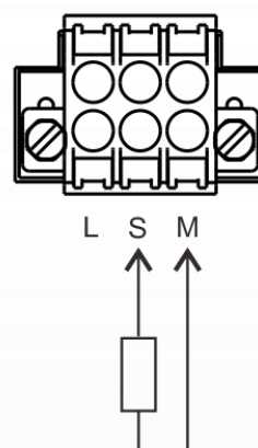
PNP输出
