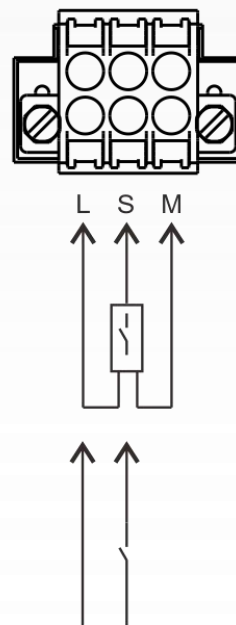
PNP输入
