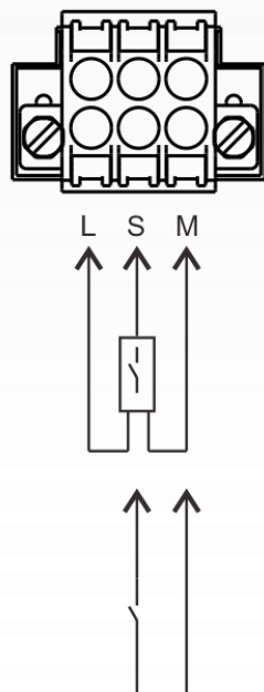
NPN输入
