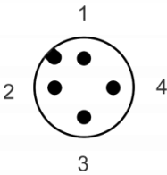
IO-Link 接口定义
