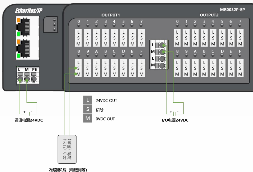
32 点输出 PNP
