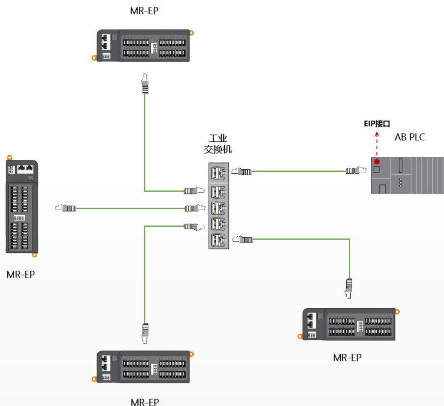
图 6-1 EtherNet/IP 星型网络拓扑结构
