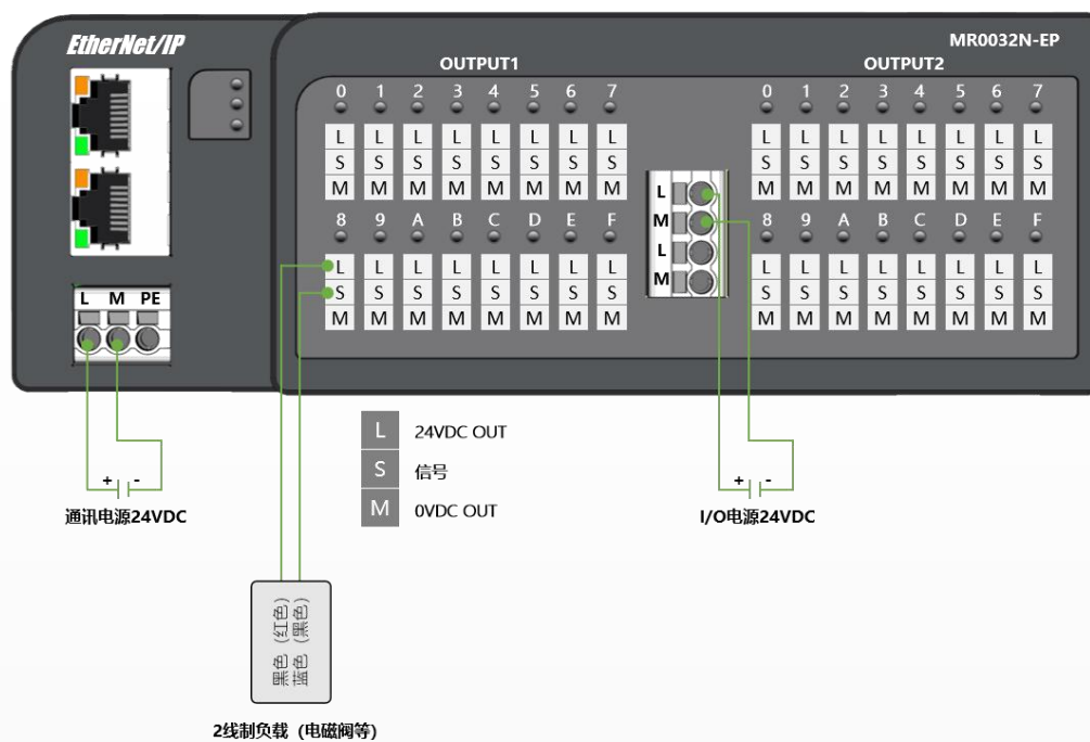
32 点输出 NPN
