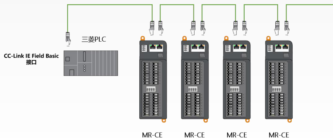
图 6-2 CC-Link IE Field Basic 菊花链网络拓扑结构
