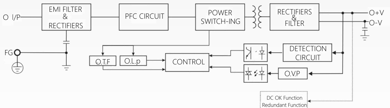
方框图
